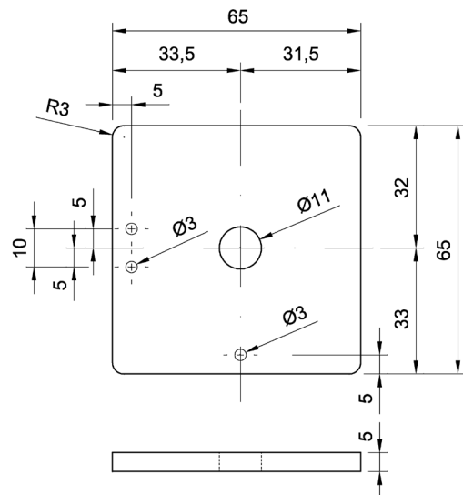
Figura 2.6: Pieza Omega. Placa de soporte 65x65x5 mm.
