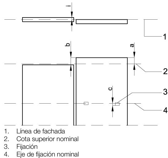
Figura 6.18: Tolerancias admisibles del montaje de los paneles.
