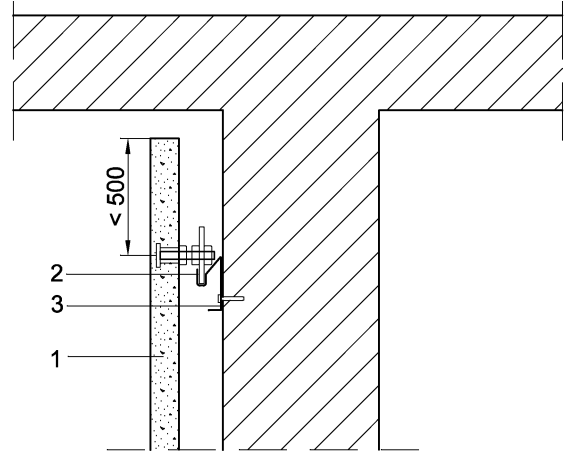
Figura 6.8: Encuentro con forjado sistema Panel ΩZ.
