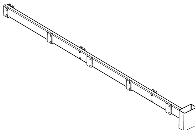
Figura 6.15: Utillaje para la colocación y nivelación de los perfiles horizontales.
