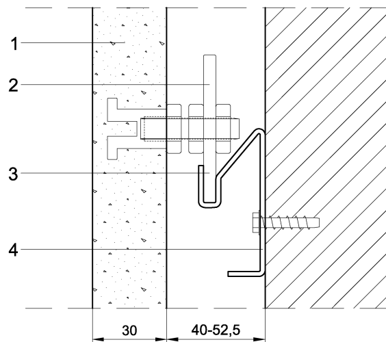
Figura 1.1: Vista del sistema Panel \Omega Z.
