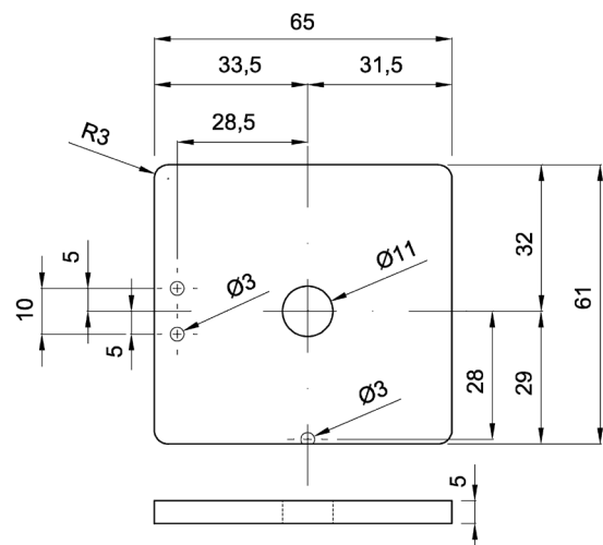
Figura 2.7: Pieza Omega. Placa de soporte 61x65x5 mm.
