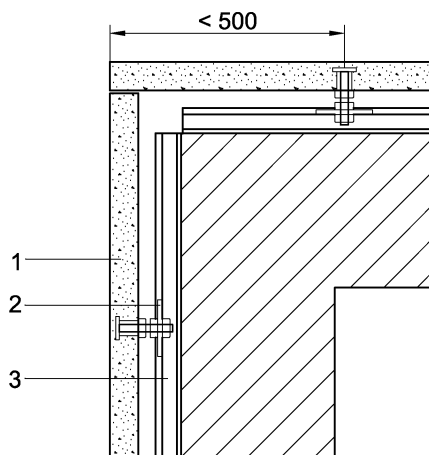
Figura 6.11: Esquina saliente sistema Panel ΩZ.
