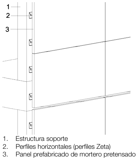
Figura 6.17: Vista del sistema Panel ΩZ.
