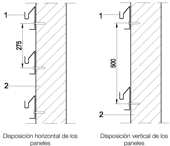
Figura 6.1: Distancia mínima entre perfiles Zeta.
