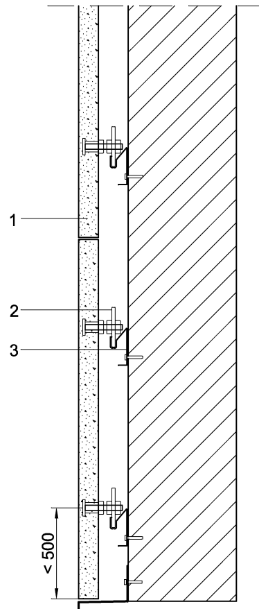
Figura 6.9: Arranque sistema Panel ΩZ.
