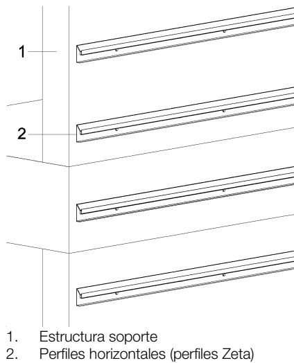
Figura 6.16: Montaje de los perfiles Zeta.
