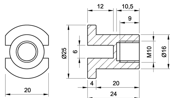
Figura 2.4: Forma y dimensiones del casquillo embebido en el panel de mortero.
