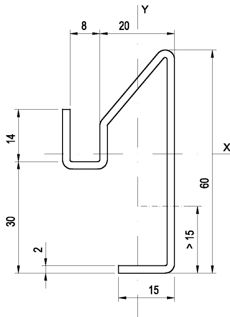
Figura 2.10: Perfil Zeta.
