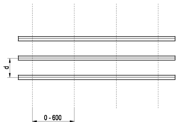
Figura 6.2: Distancia máxima entre puntos de fijación de los perfiles Zeta.
