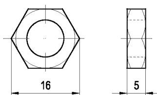
Figura 2.9: Pieza Omega. Tuerca hexagonal estrecha M10.
