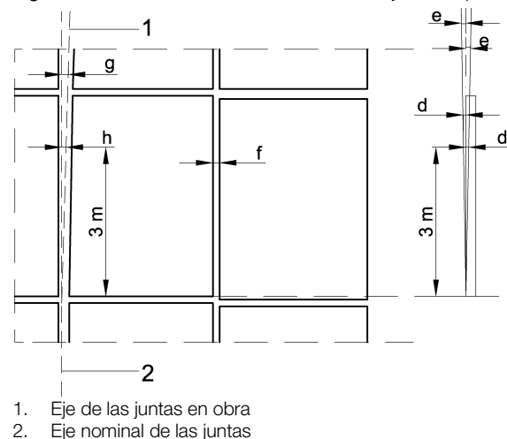
Figura 6.19: Tolerancias admisibles del montaje de los paneles.
