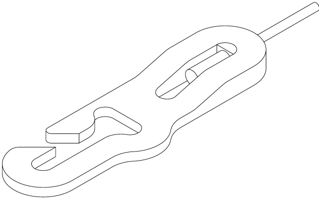
Figura 6.14: Uñas de izado de los paneles prefabricados de mortero.
